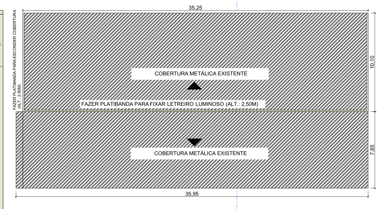
1. PLANTA COBERTURA EXISTENTE 1:200
