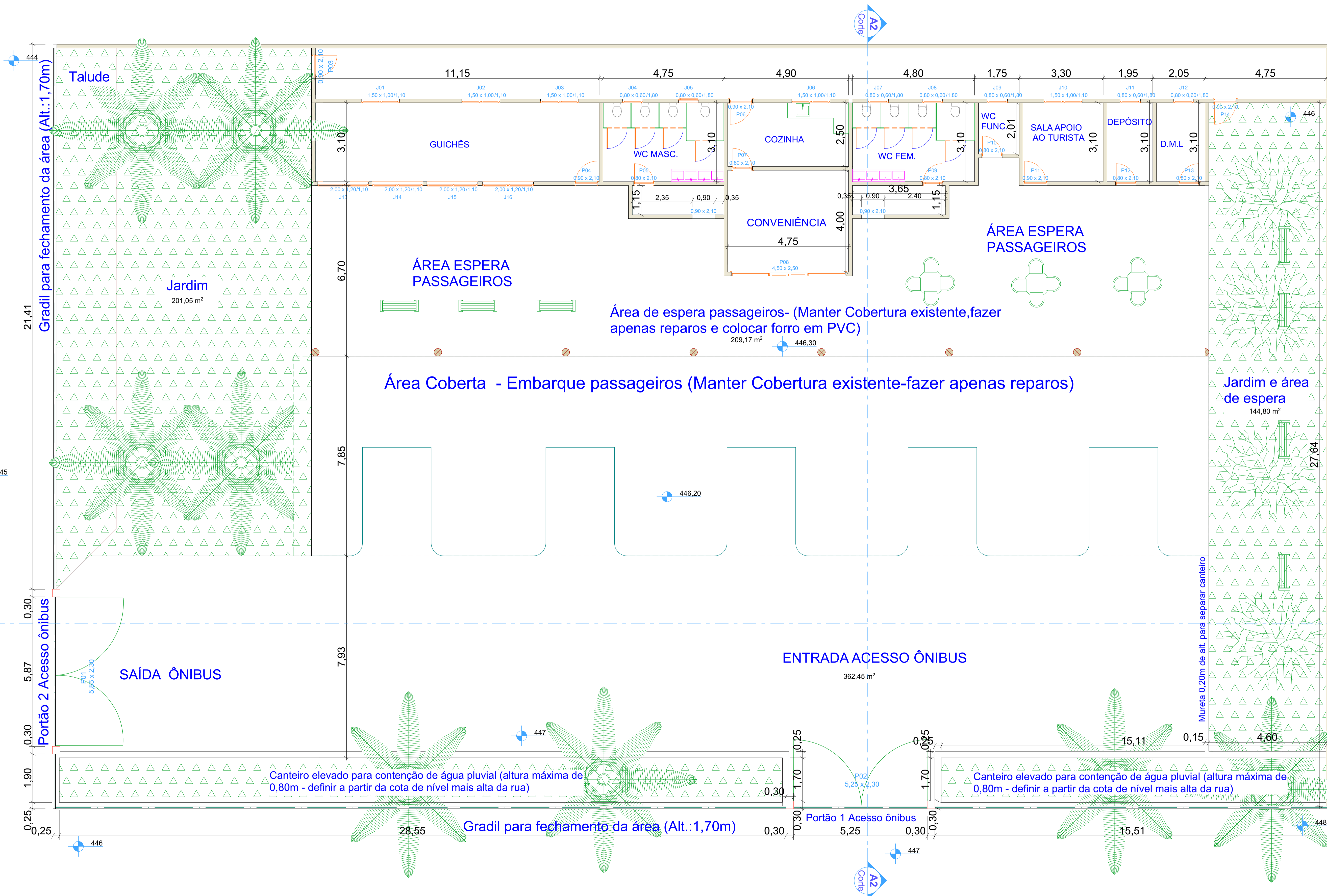
1. PLANTA COBERTURA EXISTENTE 1:200
